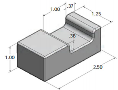
型号：DW-DT1014(W) 碳钢订货号：DW00101014 钨钢订货号：DW00102014
