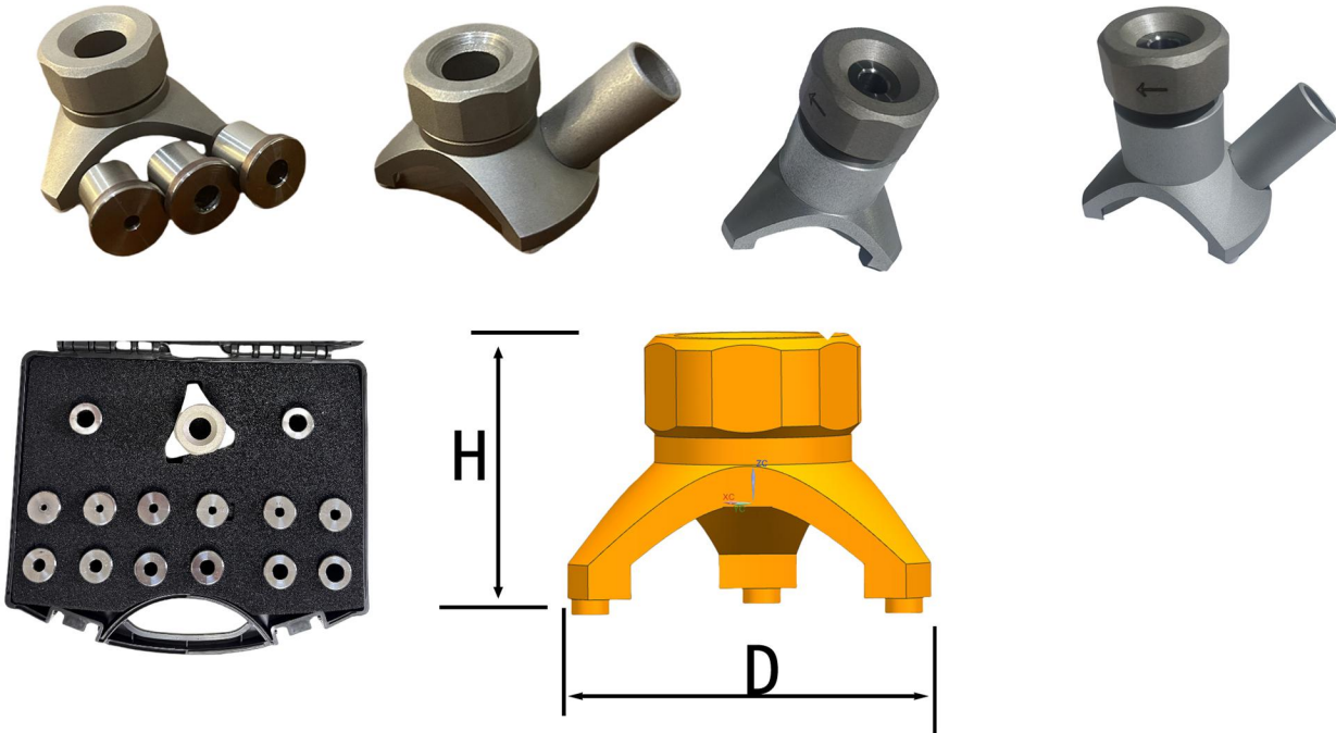
三脚架型垂直钻套套装参数表
