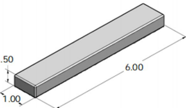
型号：DW-DT1017(W) 碳钢订货号：DW00101017 钨钢订货号：DW00102017
