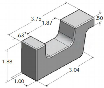
型号：DW-DT1023(W) 碳钢订货号：DW00101023 钨钢订货号：DW00102023
