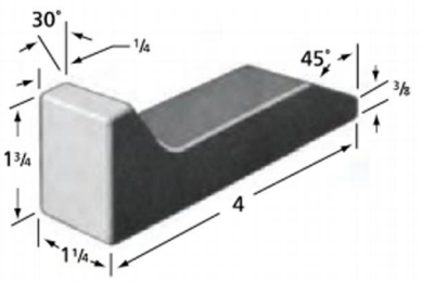
型号：DW-DT1030(W) 碳钢订货号：DW00101030 钨钢订货号：DW00102030
