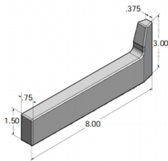
型号：DW-DT1002(W) 碳钢订货号：DW00101002 钨钢订货号：DW00102002
