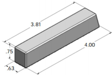
型号：DW-DT1011(W) 碳钢订货号：DW00101011 钨钢订货号：DW00102011
