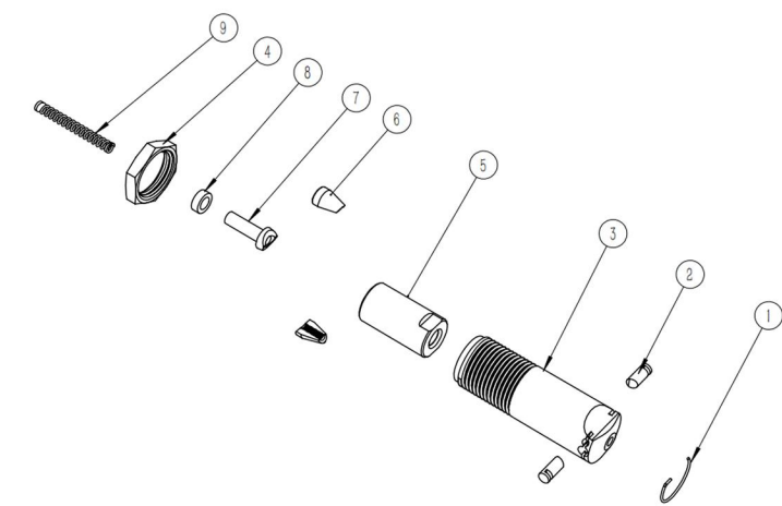
DW-H701B-456拉头分解图
