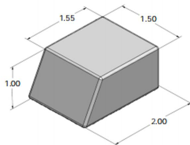
型号：DW-DT1013(W) 碳钢订货号：DW00101013 钨钢订货号：DW00102013
