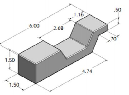
型号：DW-DT1015(W) 碳钢订货号：DW00101015 钨钢订货号：DW00102015
