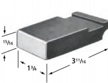
型号：DW-DT1028(W) 碳钢订货号：DW00101028 钨钢订货号：DW00102028
