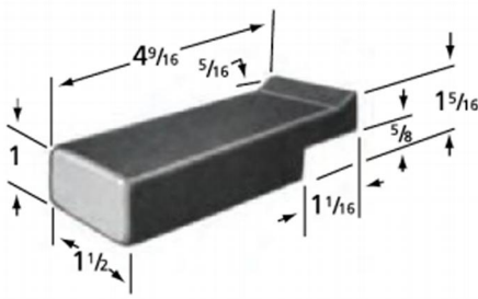
型号：DW-DT1026(W) 碳钢订货号：DW00101026 钨钢订货号：DW00102026
