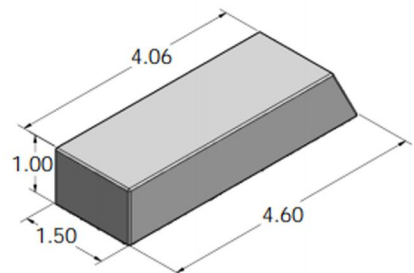
型号：DW-DT1009(W) 碳钢订货号：DW00101009 钨钢订货号：DW00102009
