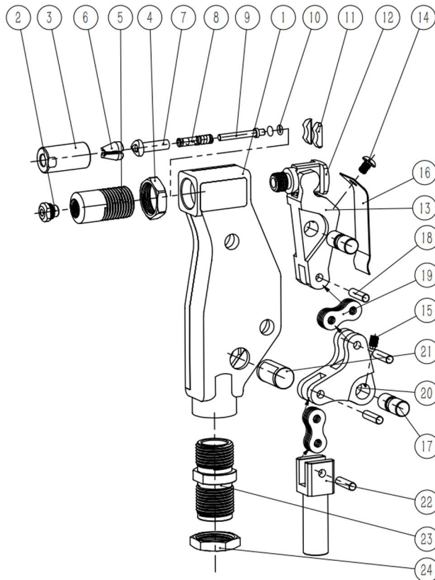
DW-H753A-456拉头分解图
