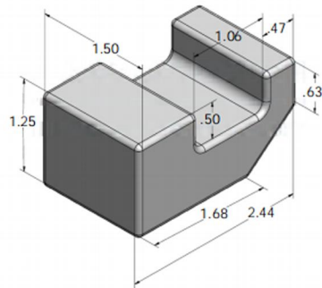
型号：DW-DT1003(W) 碳钢订货号：DW00101003 钨钢订货号：DW00102003
