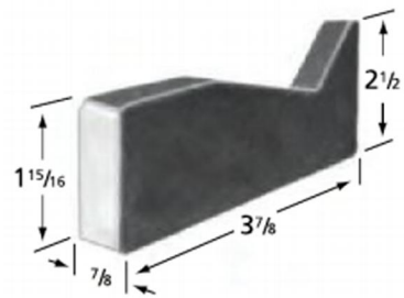
型号：DW-DT1029(W) 碳钢订货号：DW00101029 钨钢订货号：DW00102029
