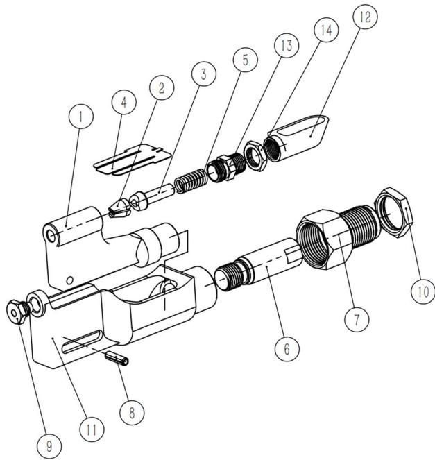
DW-H782-456拉头分解图
