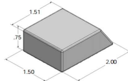
型号：DW-DT1012(W) 碳钢订货号：DW00101012 钨钢订货号：DW00102012
