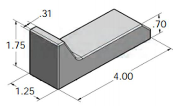
型号：DW-DT1018(W) 碳钢订货号：DW00101018 钨钢订货号：DW00102018
