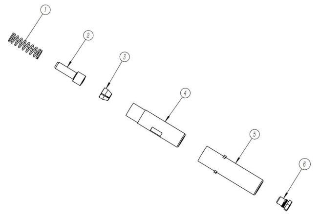
DW-H84A-8MB拉头分解图
