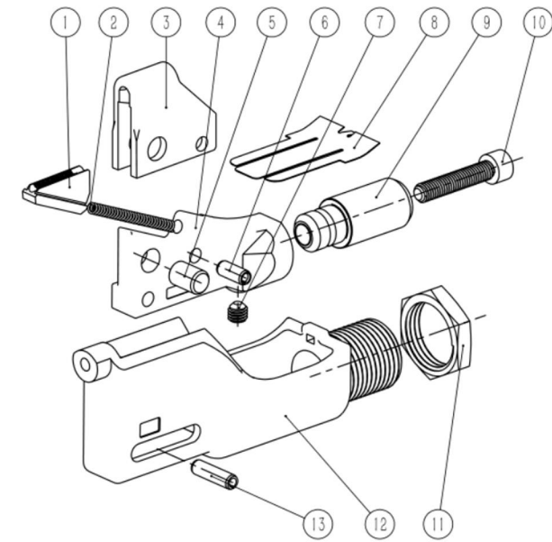
DW-H781A-456拉头分解图
