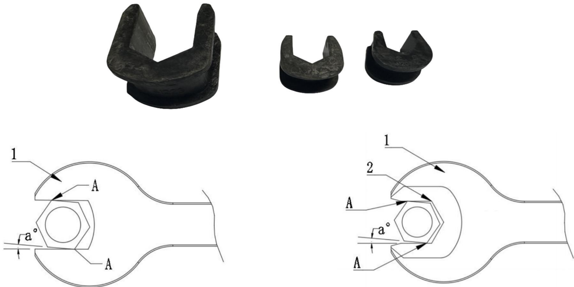
普通扳手紧固螺母示意图
