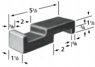
型号：DW-DT1027(W) 碳钢订货号：DW00101027 钨钢订货号：DW00102027
