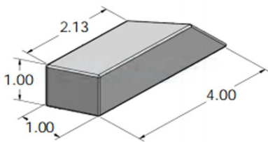
型号：DW-DT1010(W) 碳钢订货号：DW00101010 钨钢订货号：DW00102010
