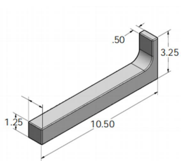
型号：DW-DT1001(W) 碳钢订货号：DW00101001 钨钢订货号：DW00102001
