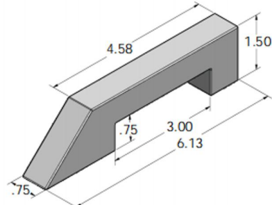
型号：DW-DT1008(W) 碳钢订货号：DW00101008 钨钢订货号：DW00102008
