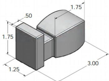
型号：DW-DT1021(W) 碳钢订货号：DW00101021 钨钢订货号：DW00102021
