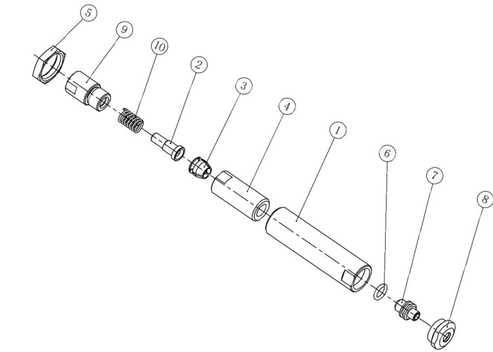
DW-H704 系列拉头分解图
