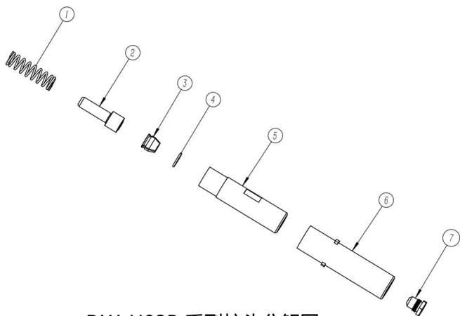
DW-H83B 系列拉头分解图
