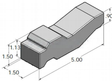
型号：DW-DT1022(W) 碳钢订货号：DW00101022 钨钢订货号：DW00102022
