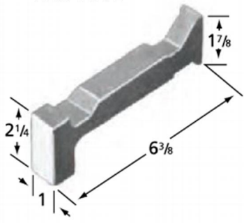
型号：DW-DT1024(W) 碳钢订货号：DW00101024 钨钢订货号：DW00102024
